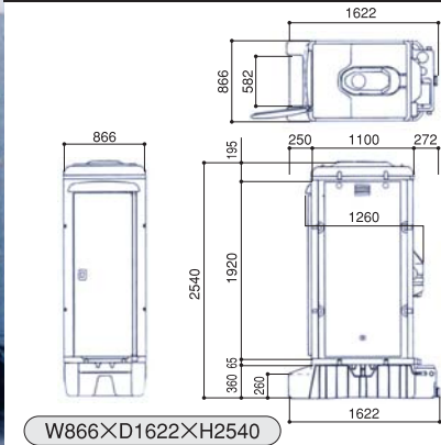
汲み取り式 (WOC-1型) ニュー軽水洗式 (WLF-1型)
