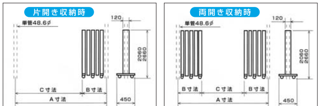
KGタイプ (基礎打ちタイプ) ●パネルゲート寸法表
