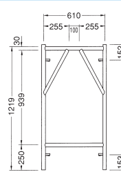
簡易枠 AB-612
