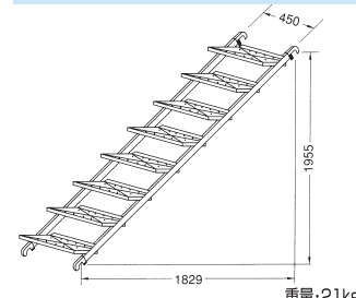
階段枠 K-3064S
