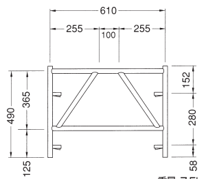
調節枠 AB-604
