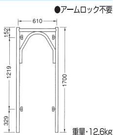
簡易枠 A-6117S(600SJ)
