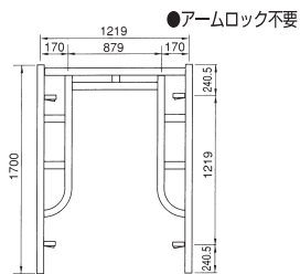
鳥居型建枠 A-4055B(1200SJ)
