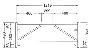
調節枠 A-417
