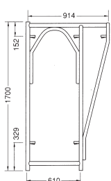
ブラケット枠 A-6117
