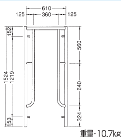
鳥居型簡易枠 A-615
