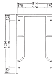
鳥居型簡易枠 A-305
