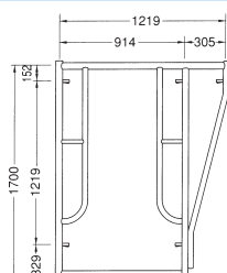
ブラケット枠 A-9117
