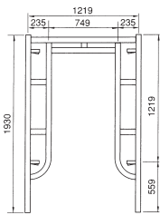
鳥居型建枠 A-4064
