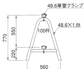
単管バリケード
