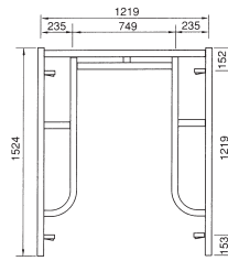
鳥居型建枠 A-405
