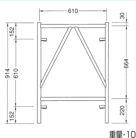
簡易枠 AB-609
