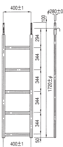
単管バリケード
