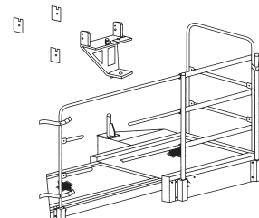
レインボー・ステージ ターン型コーナー用
