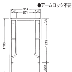
鳥居型建枠 A-3055A(900SJ)
