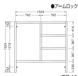
梯子型建枠 A-2(1500SJ)
