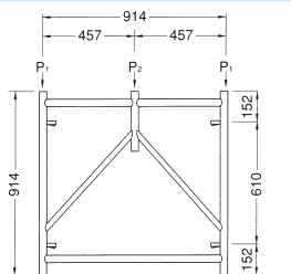
支保工ブラケット枠 AB-909
