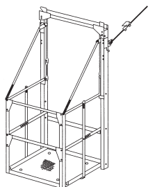
アルミハンガー 075・105・150
