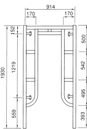
鳥居型建枠 A-3064
