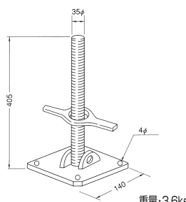
自在ジャッキベース
