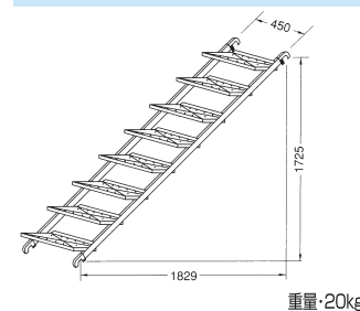
階段枠 K-3055S
