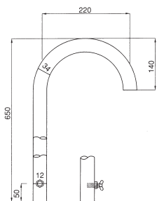
モンキーヘッド
