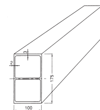
アルミ大引材175
