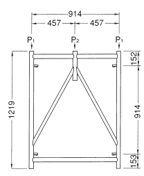
鳥居型建枠 AB-912
