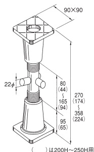
アルミハンガー 075・105・150
