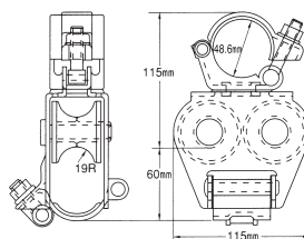
レインボー・ステージ フィックス型
