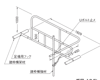
階段枠 K-3055S
