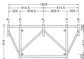
支保工ブラケット枠 AB-1809
