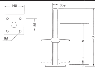
ジャッキベース(ミゾ切)
