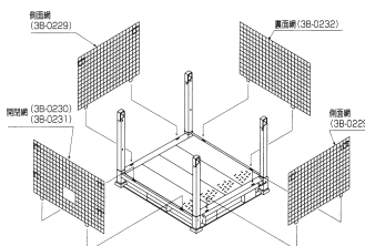
マルチパレットMPS
